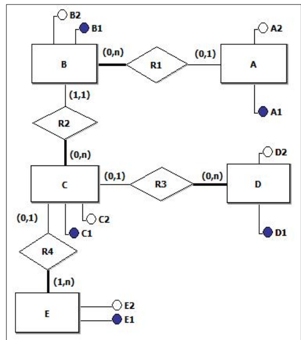
Figura 8 - DER
