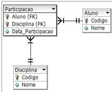
Figura 7(a) - DER
